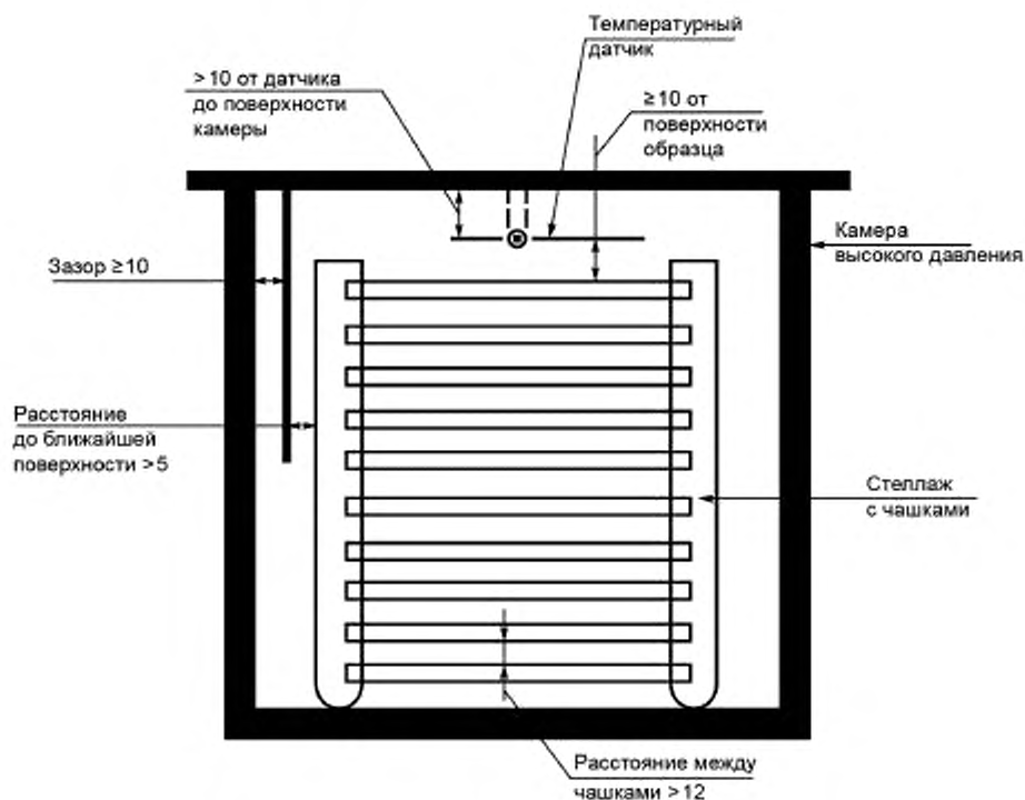
Рисунок 2 — Схема камеры высокого давления
