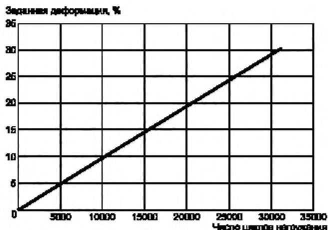
Рисунок 2 — Условия изменения заданной деформации при проведении испытаний
