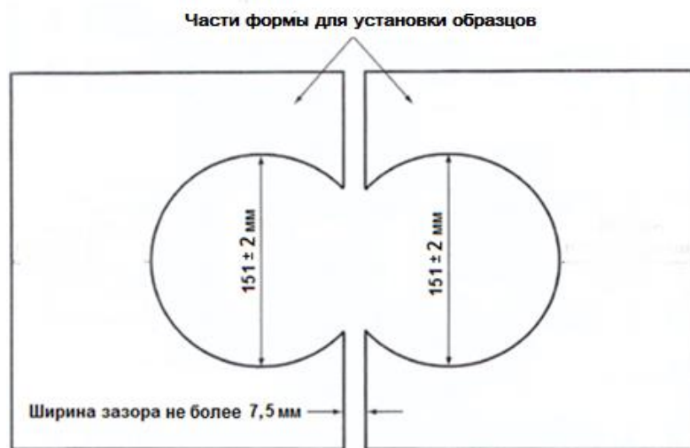
Рисунок А.2 – Схема монтажа цилиндрических образцов
